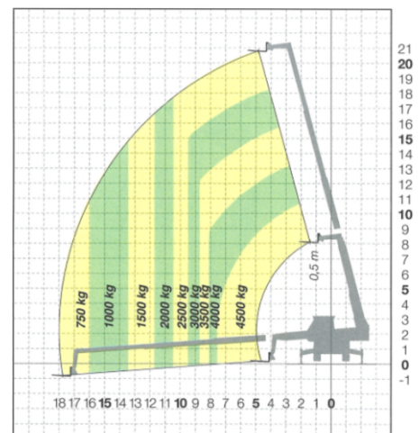
ROTO 45.21 MCSS MIT LASTGABELN AUF ABSTÜTZUNGEN - 360°
